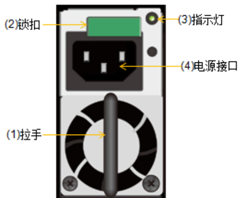
图3-31 DSU2624 电源模块正视图
