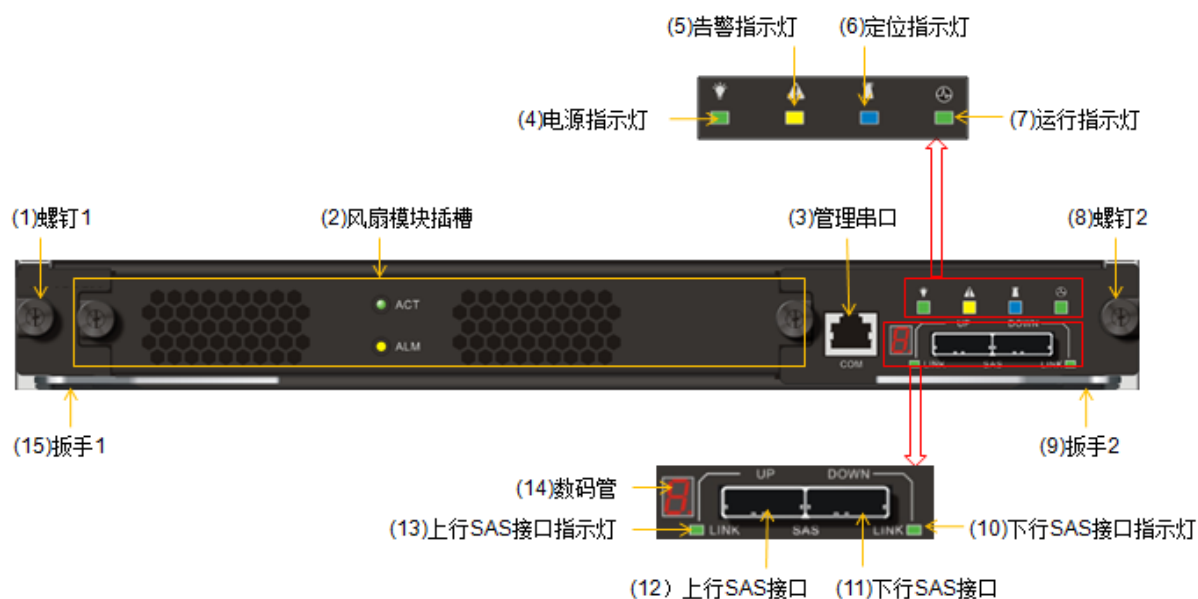
图3-25 DSU1616 EP 正视图
