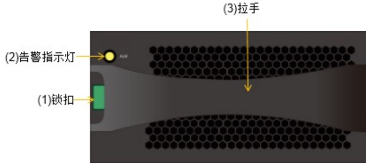
图3-30 DSU2624 风扇模块正视图
