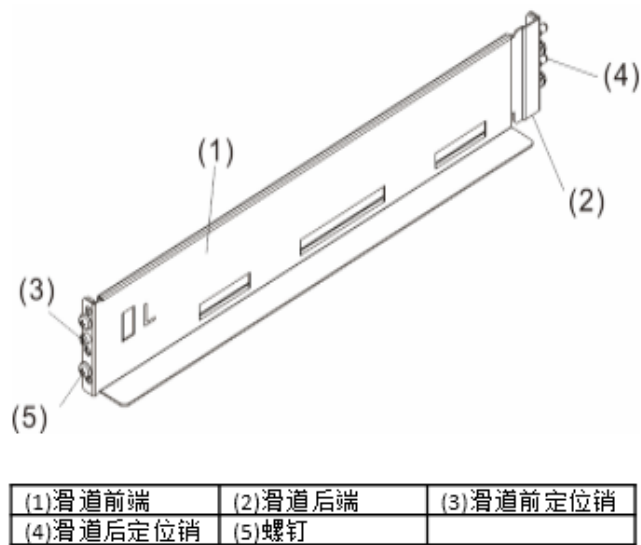
图4-5 带定位销托架式滑道（左侧滑道）示意图
