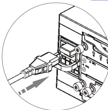
图4-26 安装电源线示意图（二）
