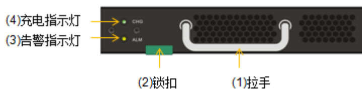
图3-14 4U SPU 电池模块正视图
