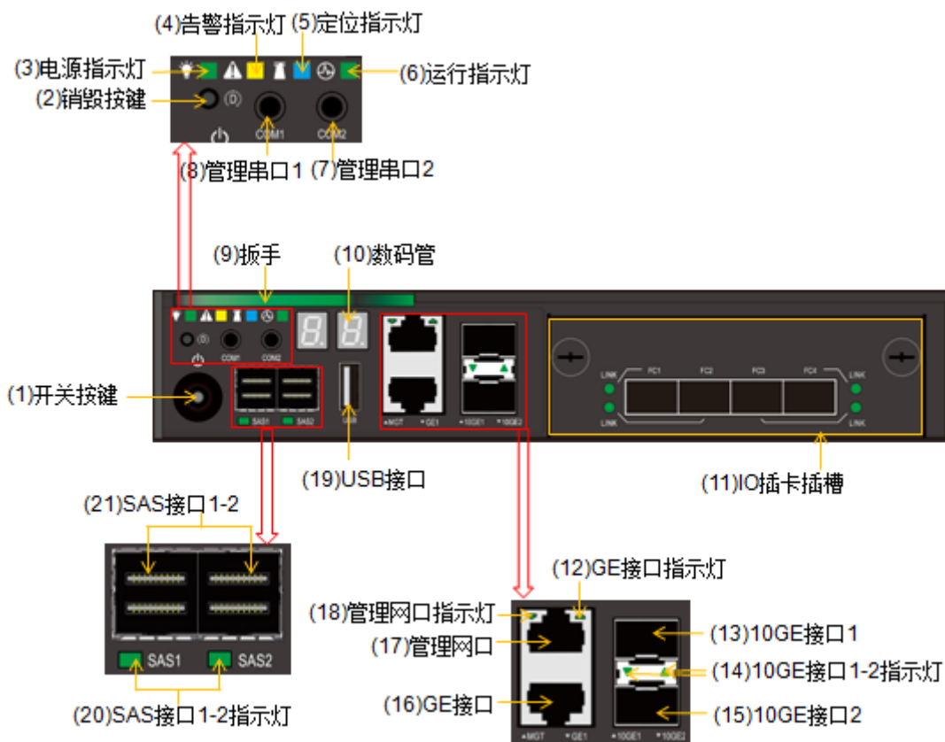
图3-6 2U SPU 的 SP 正视图（三）
