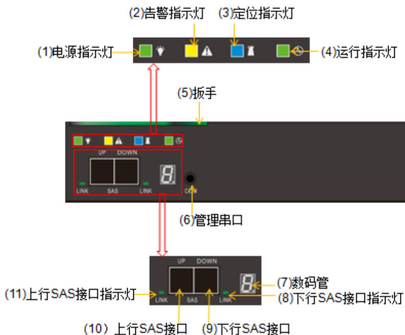
图3-20 DSU2625 的 EP 正视图
