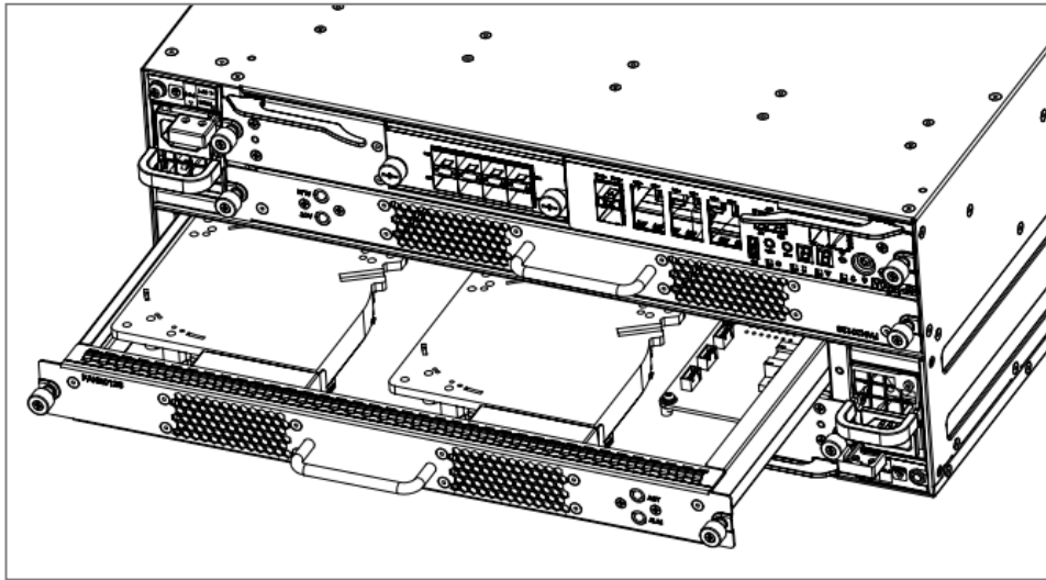
图6-10 安装/拆卸 MS2500G2-16A 标准版 SPU 风扇模块示意图
