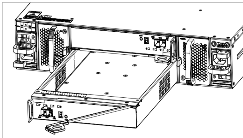
图6-5 安装/拆卸 DSU2625 EP 示意图
