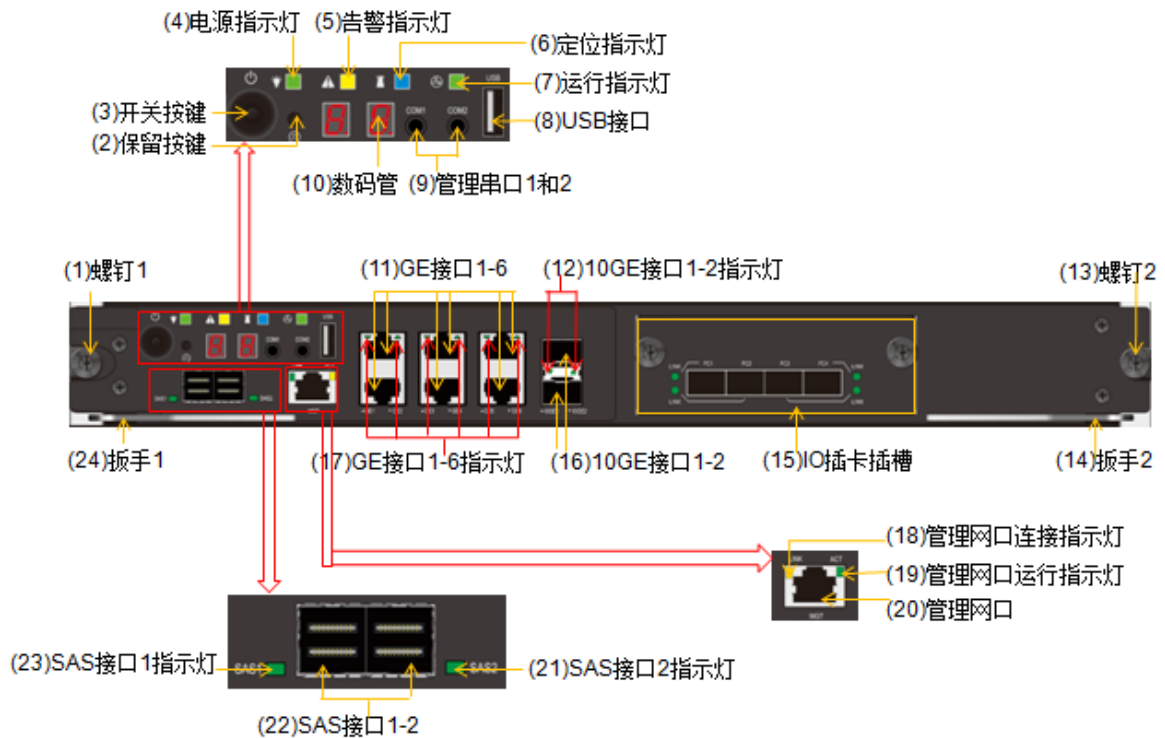
图3-12 4U SPU 的 SP 正视图
