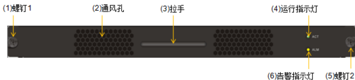
图3-13 4U SPU 风扇模块正视图
