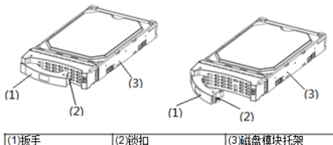
图6-29 3.5 英寸磁盘模块 B 示意图
