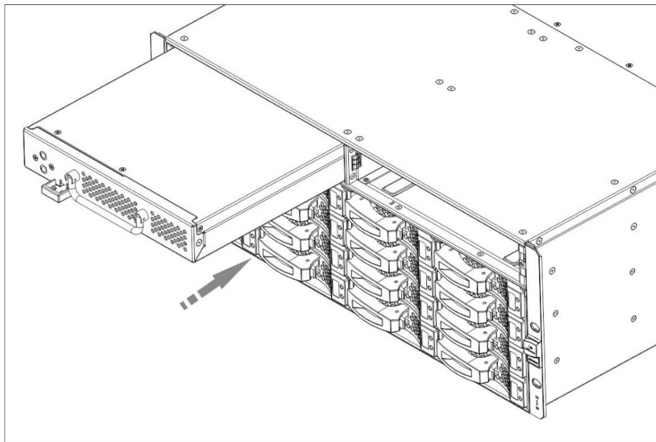
图4-13 安装 4U SPU 电池模块示意图
