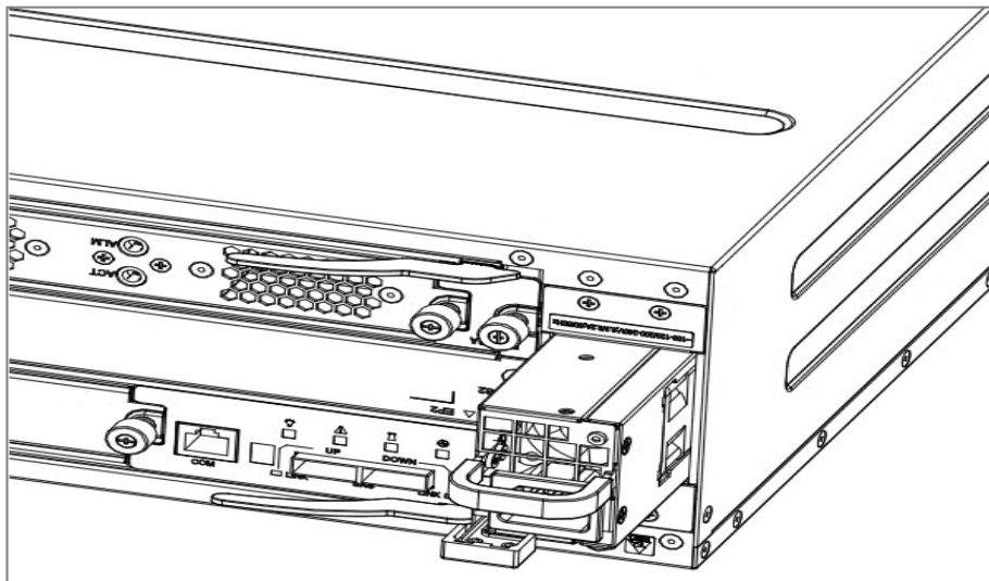
图6-16 安装/拆卸 DSU1616 电源模块示意图
