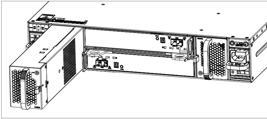
图6-13 安装/拆卸 DSU2625 风扇模块示意图
