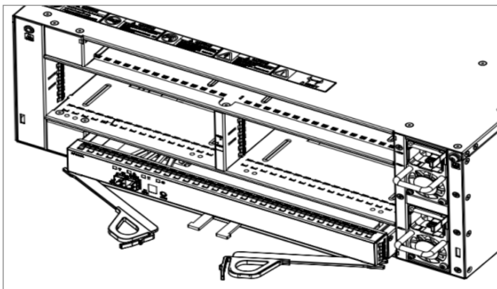
图6-7 安装/拆卸 DSU2624 EP 示意图
