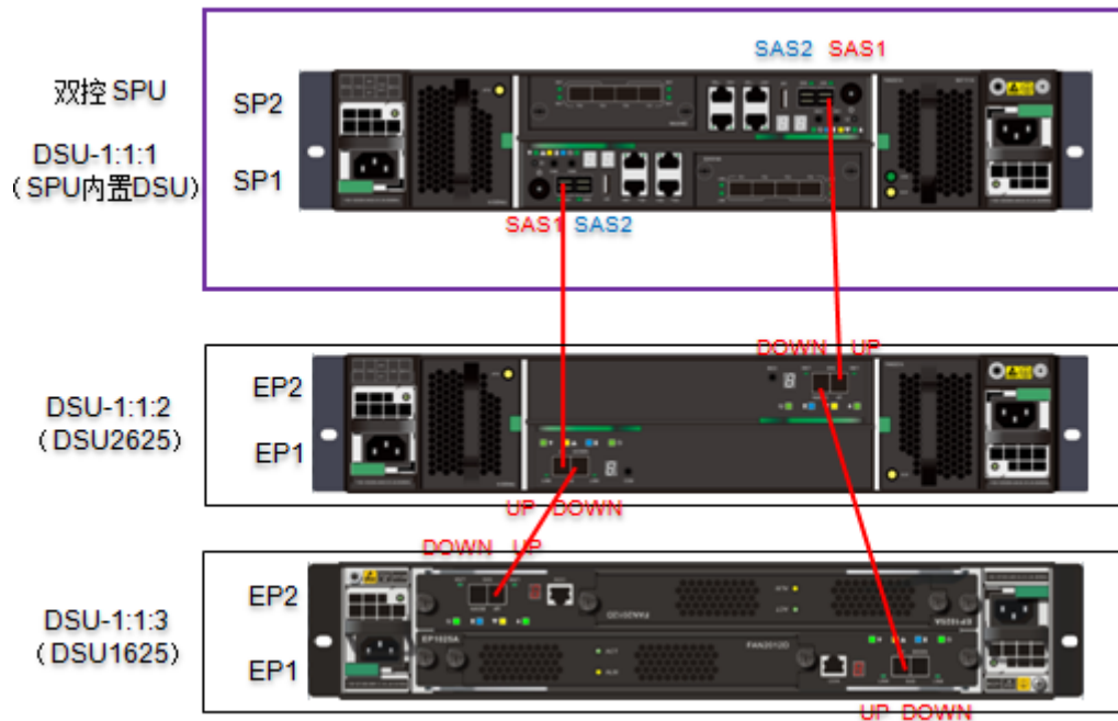
图4-37 SAS1 接口上 SAS 线缆安装示意图
