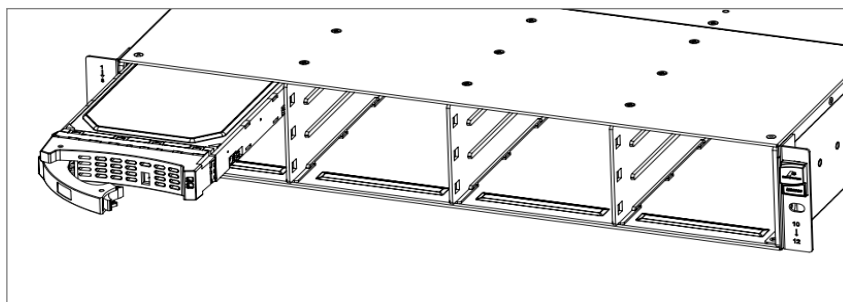
图6-32 安装 3.5 英寸磁盘模块 B 示意图
