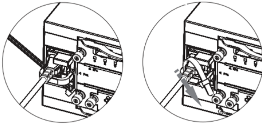
图4-27 电源线捆扎示意图
