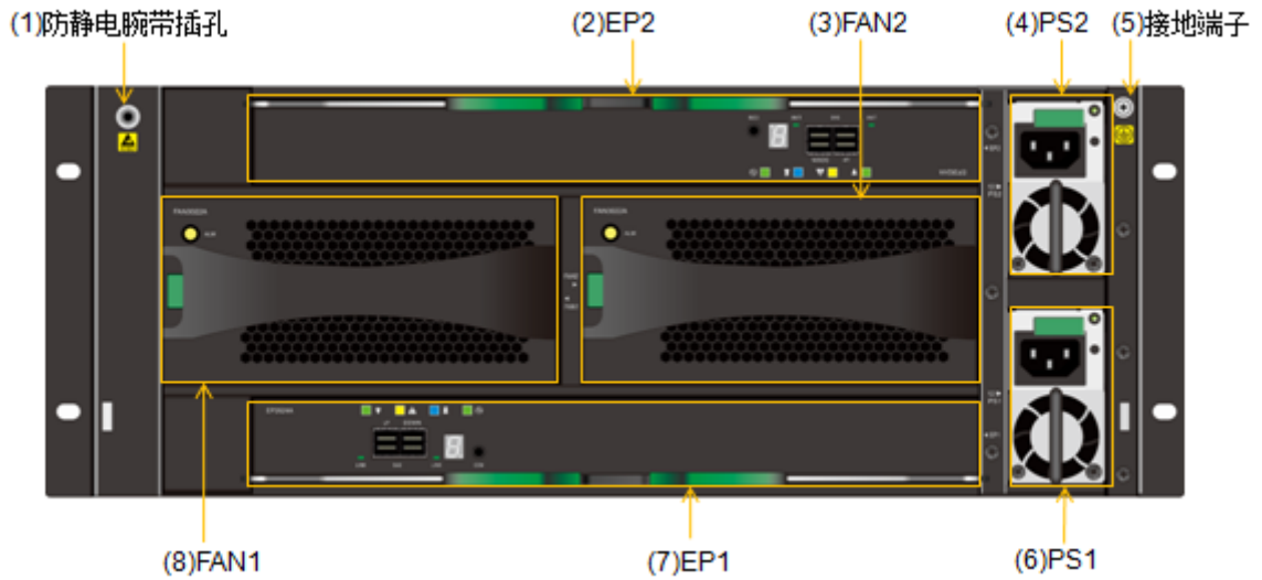
图3-28 DSU2624 后正视图
