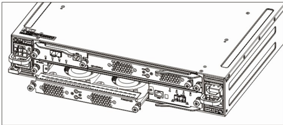
图6-12 安装/拆卸 DSU1625 风扇模块示意图
