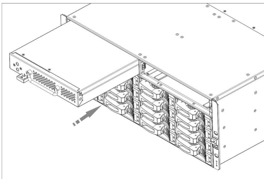
图6-11 安装/拆卸 MS2500G2-16A 标准版 SPU 电池模块示意图
