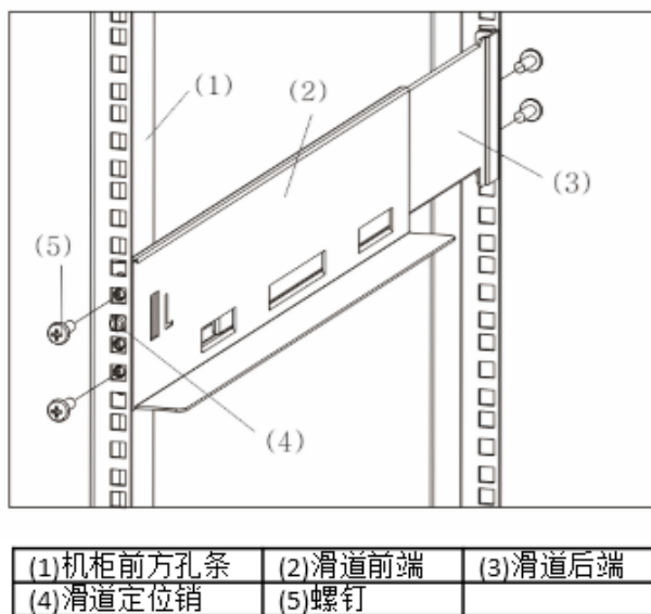
图4-9 安装带定位销的托架式左侧滑道示意图
