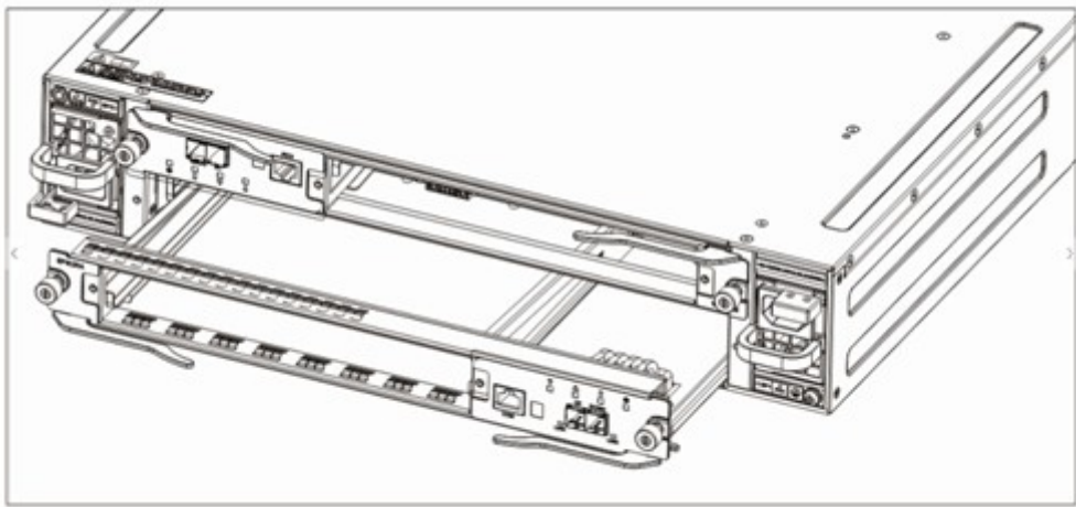
图6-4 安装/拆卸 DSU1625 EP 示意图
