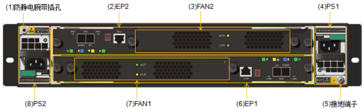
图3-17 DSU1625 后正视图
