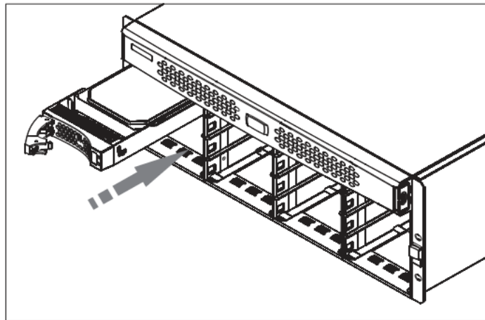
图6-28 安装 3.5 英寸磁盘模块 A 示意图
