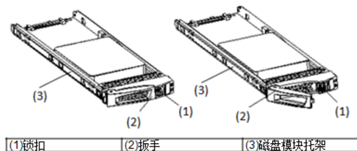
图6-19 2.5 英寸磁盘模块 A 示意图
