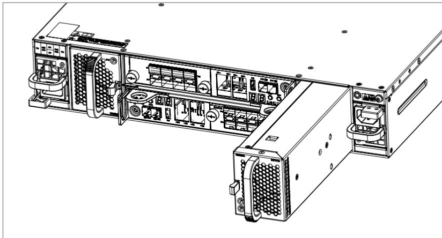
图4-12 安装 2U SPU 风扇模块（含电池模块）示意图
