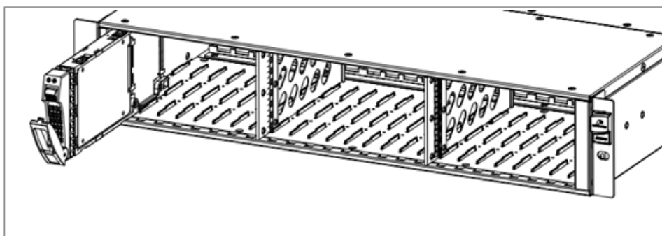
图6-24 安装 2.5 英寸磁盘模块 B 示意图
