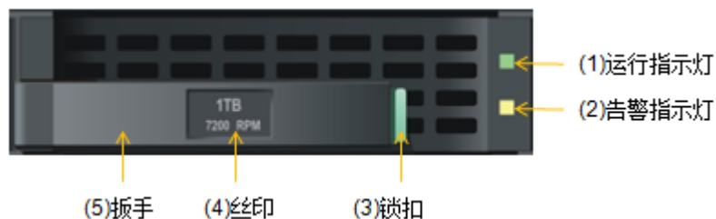
图3-37 3.5 英寸磁盘模块前面板
