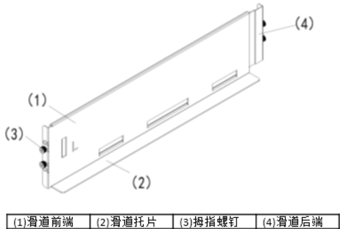
图4-4 带拇指螺钉托架式滑道（左侧滑道）示意图
