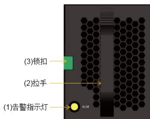
图3-22 DSU2625 风扇模块正视图
