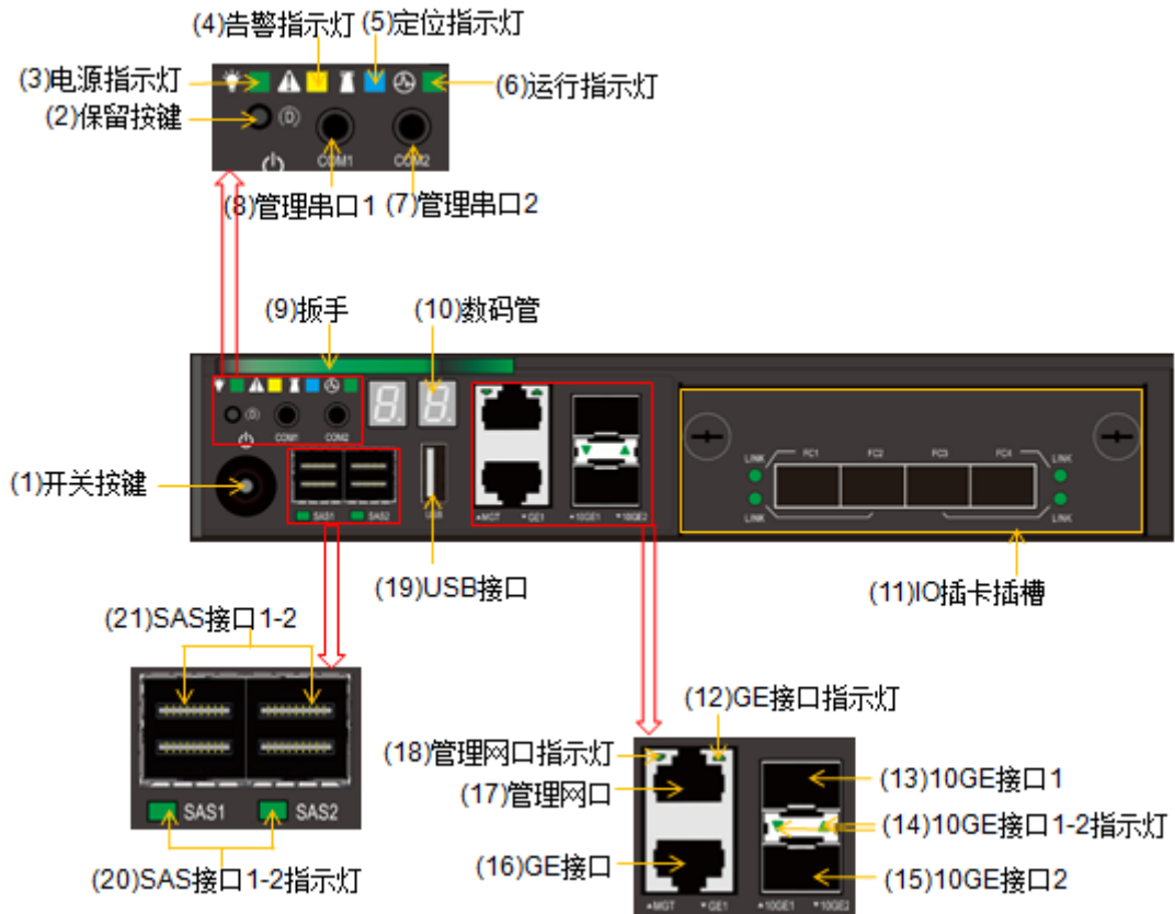
图3-5 2U SPU 的 SP 正视图（二）
