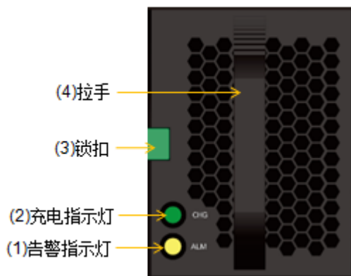
图3-8 2U SPU 风扇模块（含电池模块）正视图
