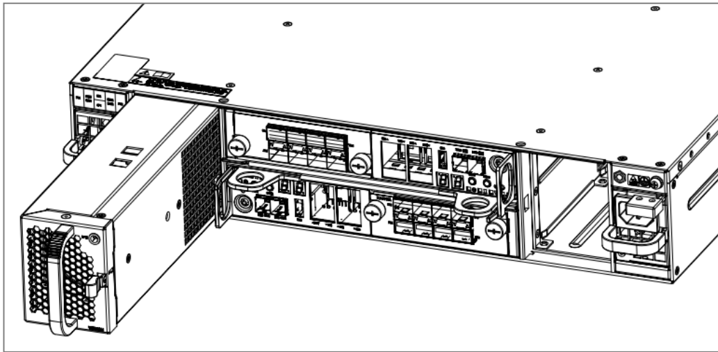
图6-8 安装/拆卸 MS2500G2-12S SPU 风扇模块（无电池模块）示意图
