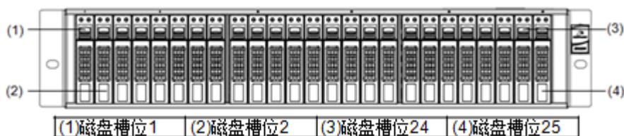
图6-23 2.5 英寸磁盘模块 B 槽位编号示意图
