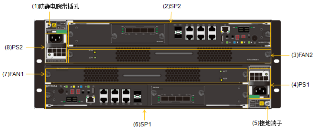
图3-11 4U SPU 后正视图
