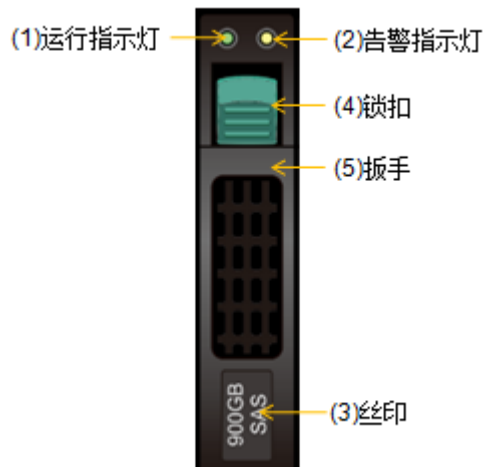
图3-34 2.5 英寸磁盘模块 B 前面板
