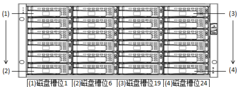
图6-31 3.5 英寸磁盘模块 B 槽位编号示意图（二）
