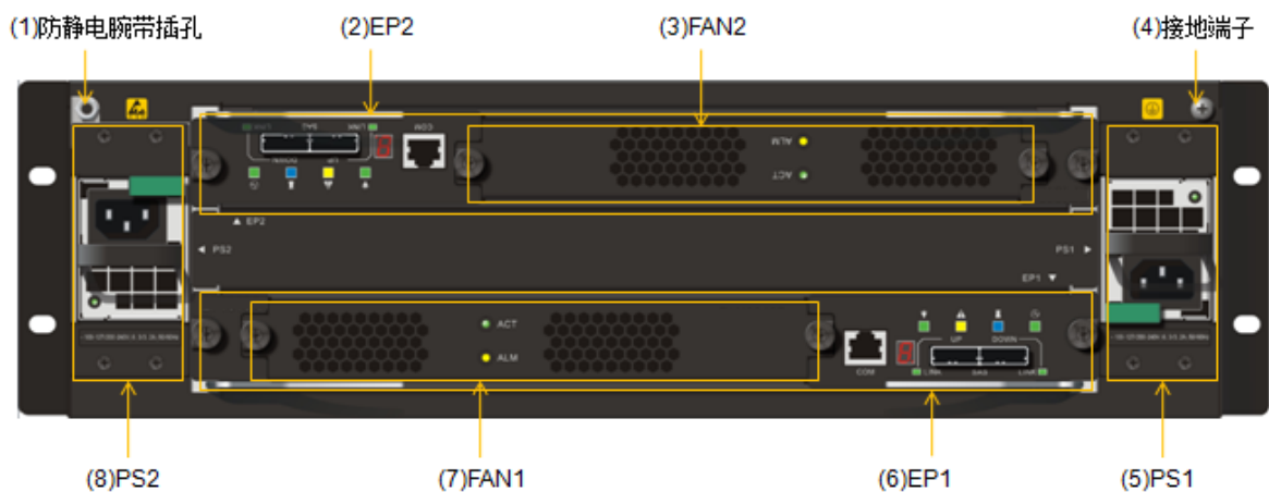
图3-24 DSU1616 后正视图
