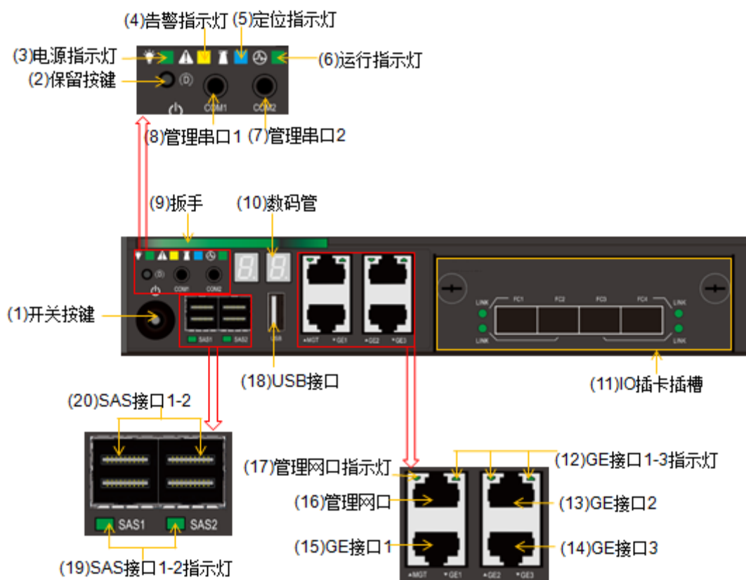
图3-4 2U SPU 的 SP 正视图（一）
