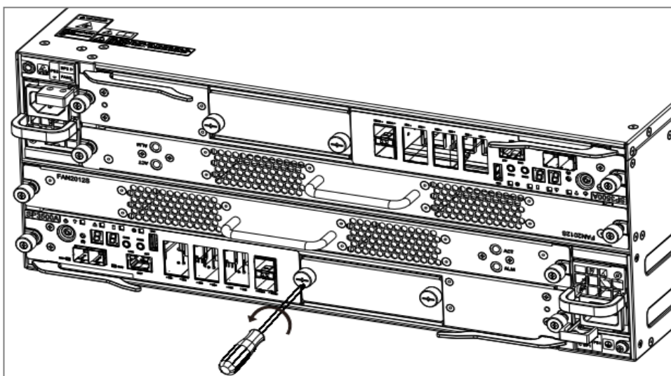
图6-18 拆卸 IO 插卡假面板示意图
