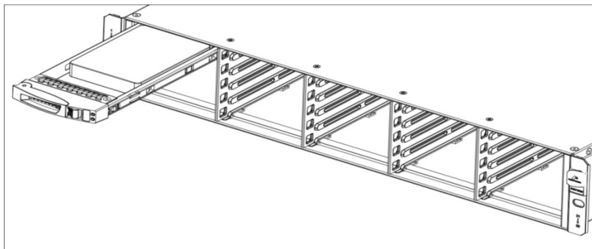
图6-21 安装 2.5 英寸磁盘模块 A 示意图
