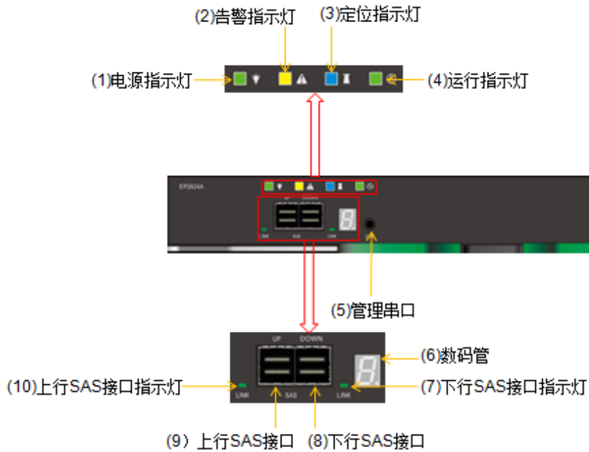
图3-29 DSU2624 EP 正视图
