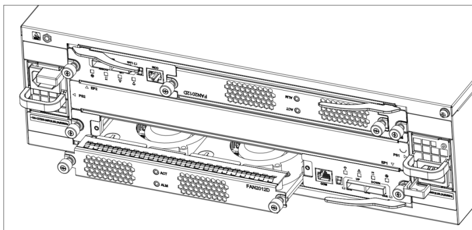
图6-14 安装/拆卸 DSU1616 风扇模块示意图
