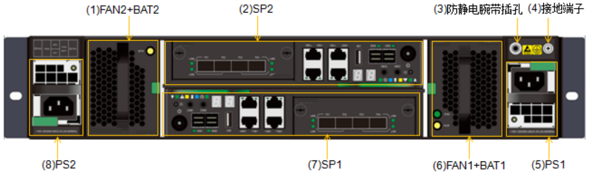
图3-3 MS2500G2-12S SPU 后正视图
