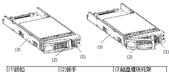
图6-22 2.5 英寸磁盘模块 B 示意图
