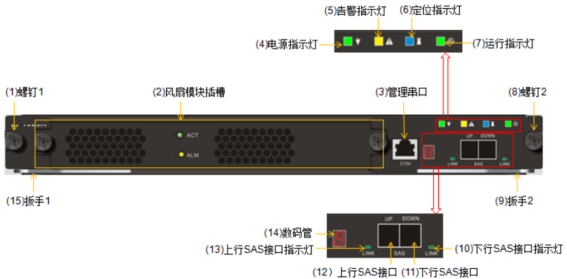
图3-19 DSU1625 EP 正视图
