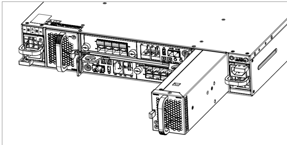
图6-9 安装/拆卸 MS2500G2-12S SPU 风扇模块（含电池模块）示意图
