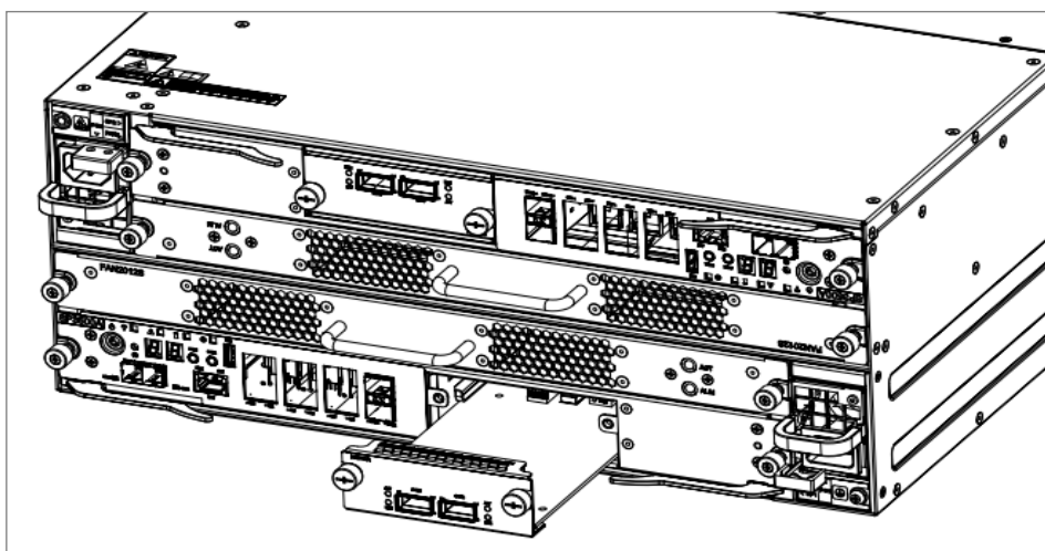
图6-17 安装/拆卸 IO 插卡模块示意图
