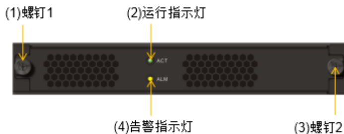
图3-26 DSU1616 风扇模块正视图
