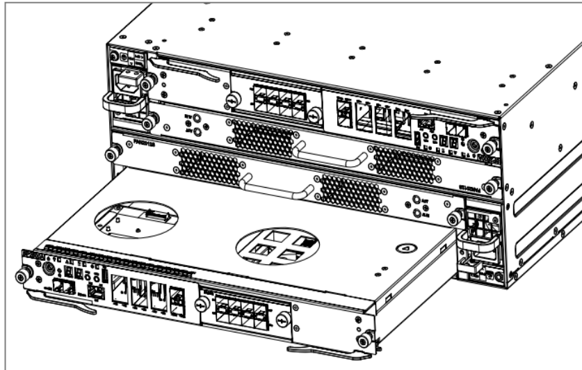
图6-3 安装/拆卸 MS2500G2-16A 标准版 SP 示意图
