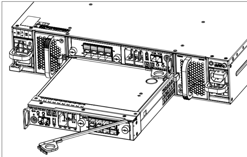
图6-2 安装/拆卸 MS2500G2-12S SP 示意图
