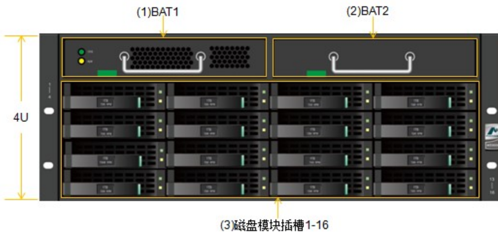
图3-10 4U SPU 前正视图（不带面板）
