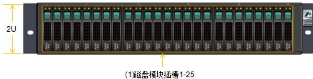
图3-2 2U SPU 前正视图（二）
