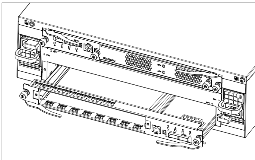
图6-6 安装/拆卸 DSU1616 EP 示意图
