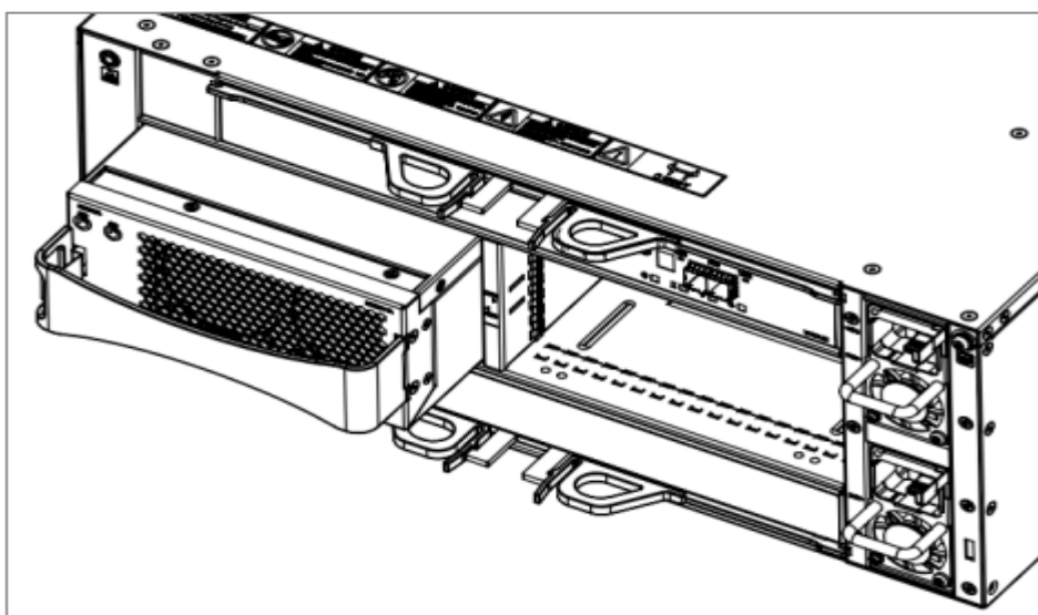
图6-15 安装/拆卸 DSU2624 风扇模块示意图
